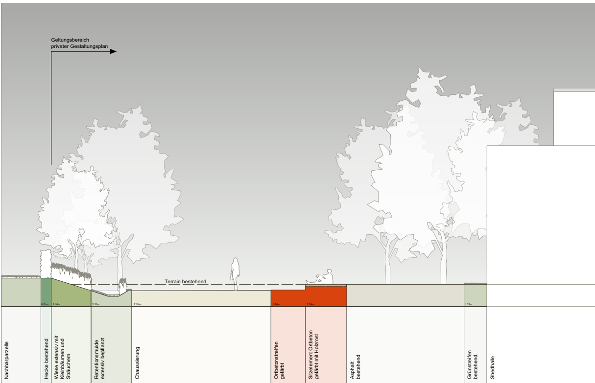
Schnitt B-B' massstablos
